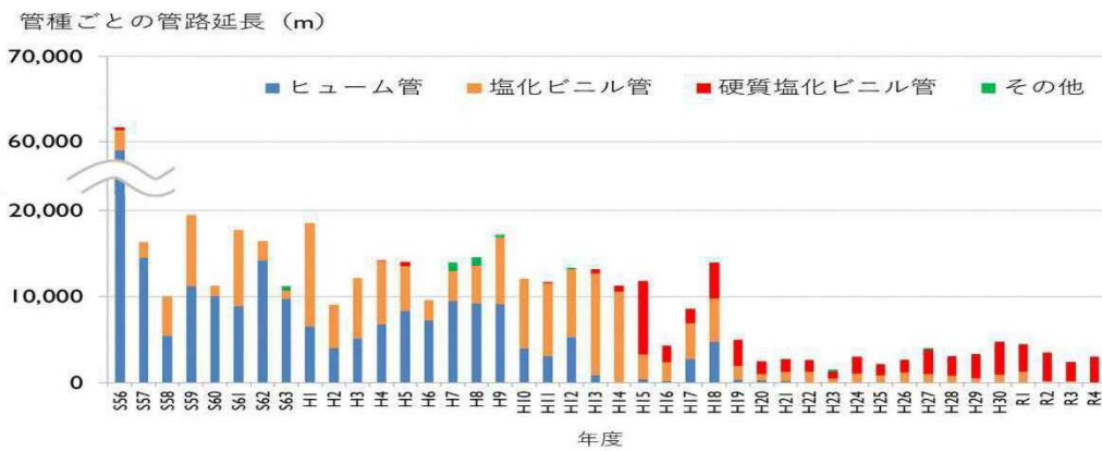
図 17 管種ごとの管路延長 (p 22)
