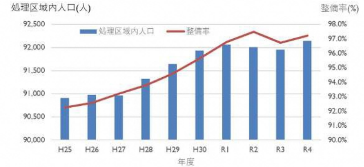
図 14 処理区域内人口と整備率の推移
