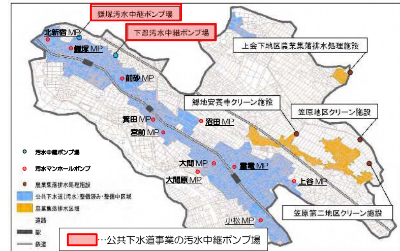
図 19 污水ポンプ場施設位置図（污水）
