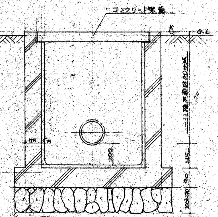
排水槽详细图
