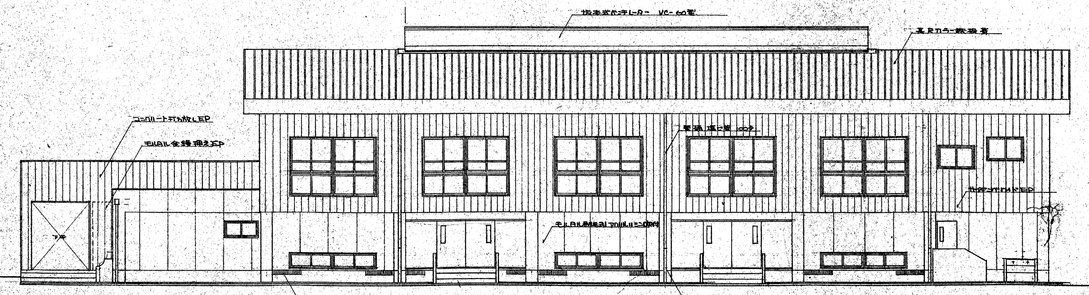
南立面図 S=1:100
