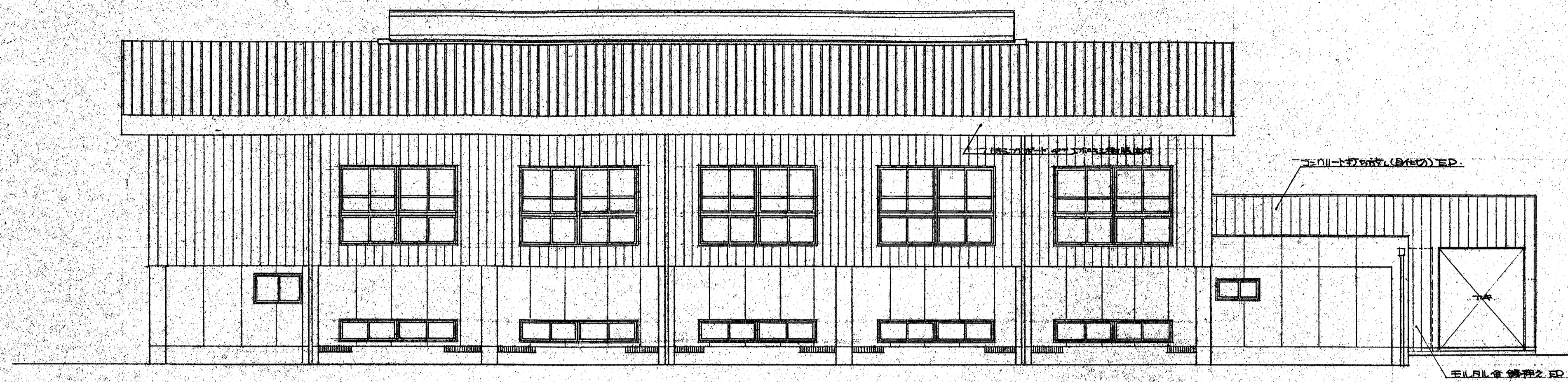
北立面図 S=1:100
