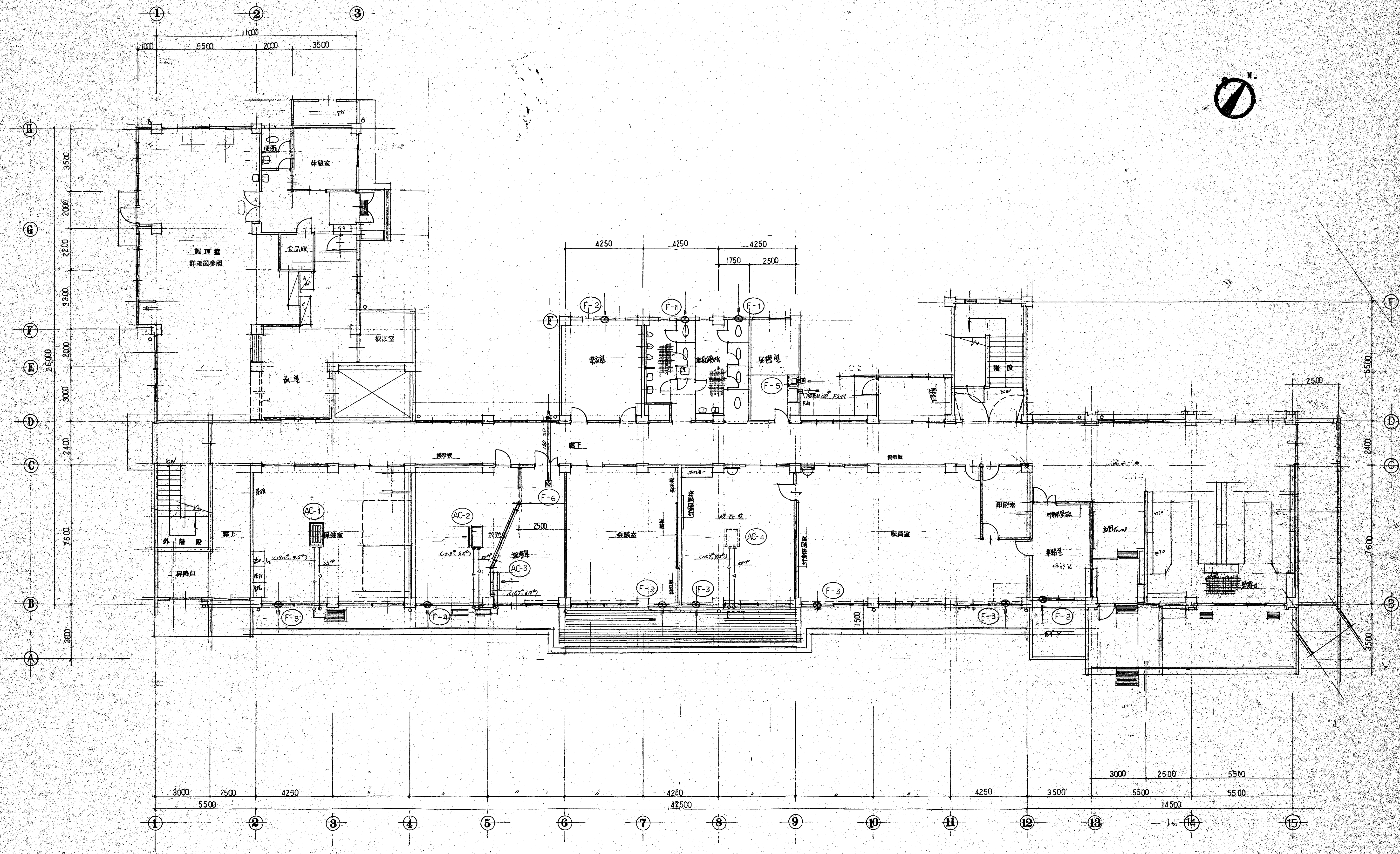
1階平面図
