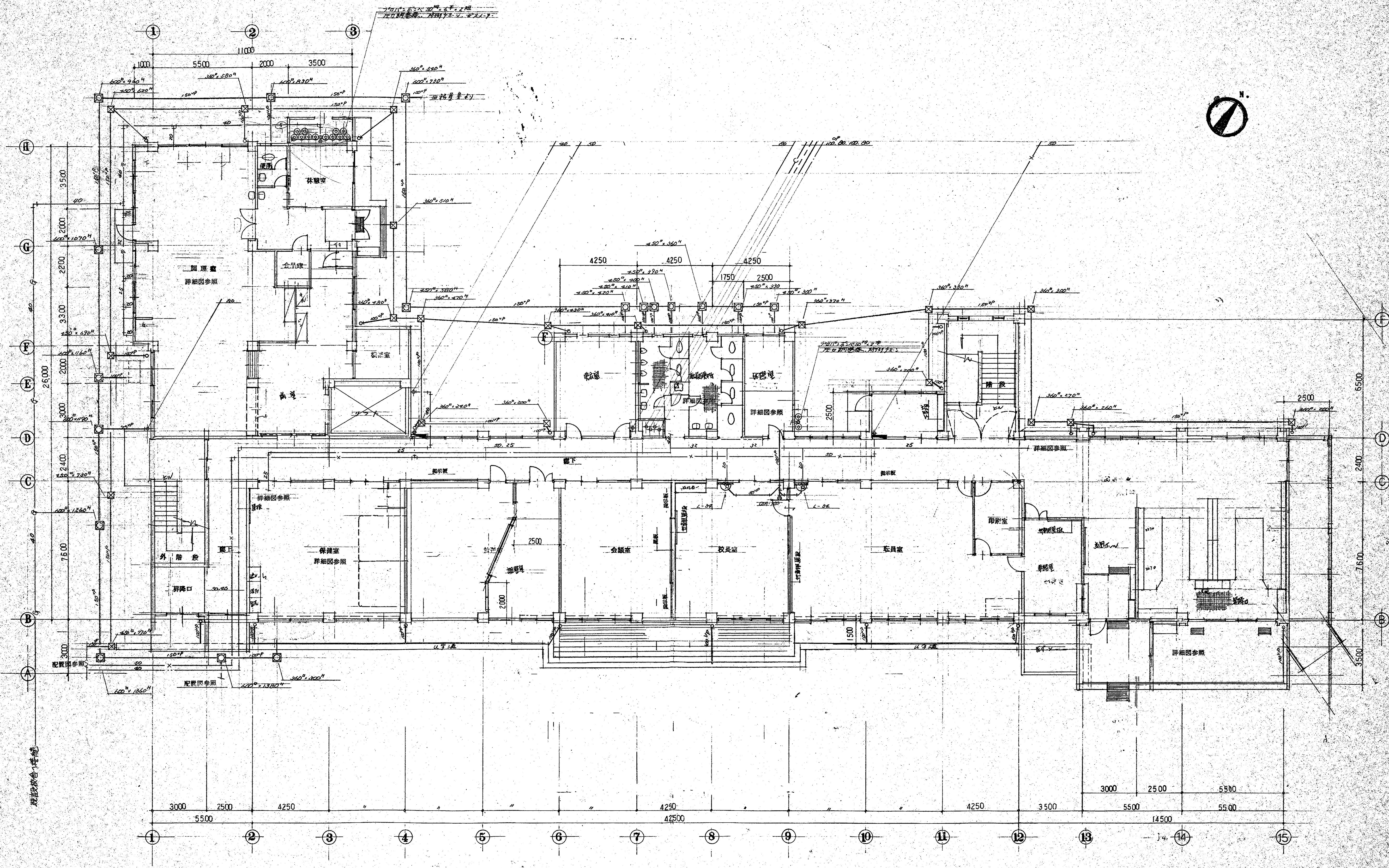
1 階平面圖
