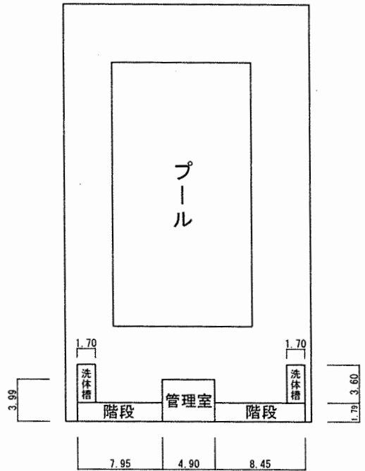
2階
