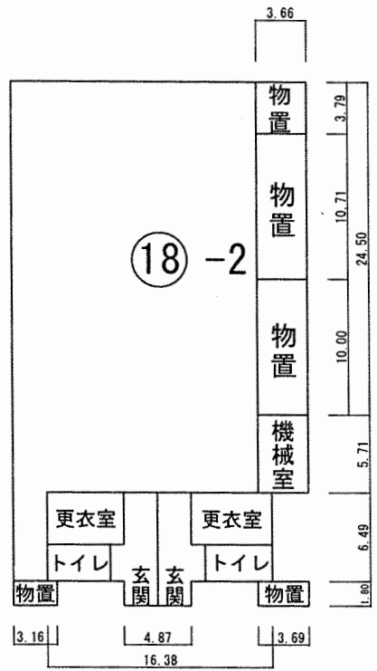
1階
