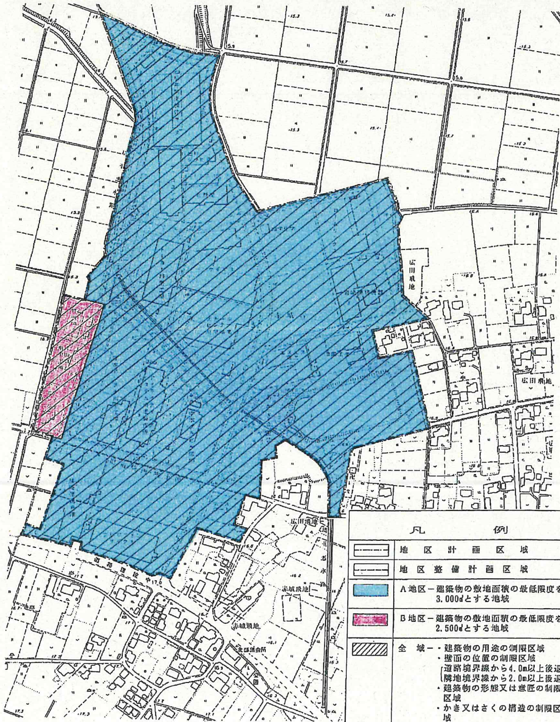
〔地区整備計画図〕
