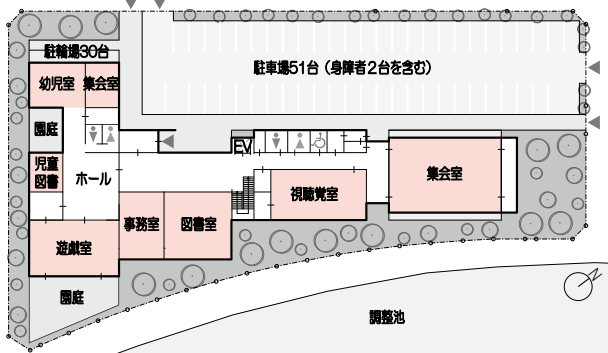
1階平面図
