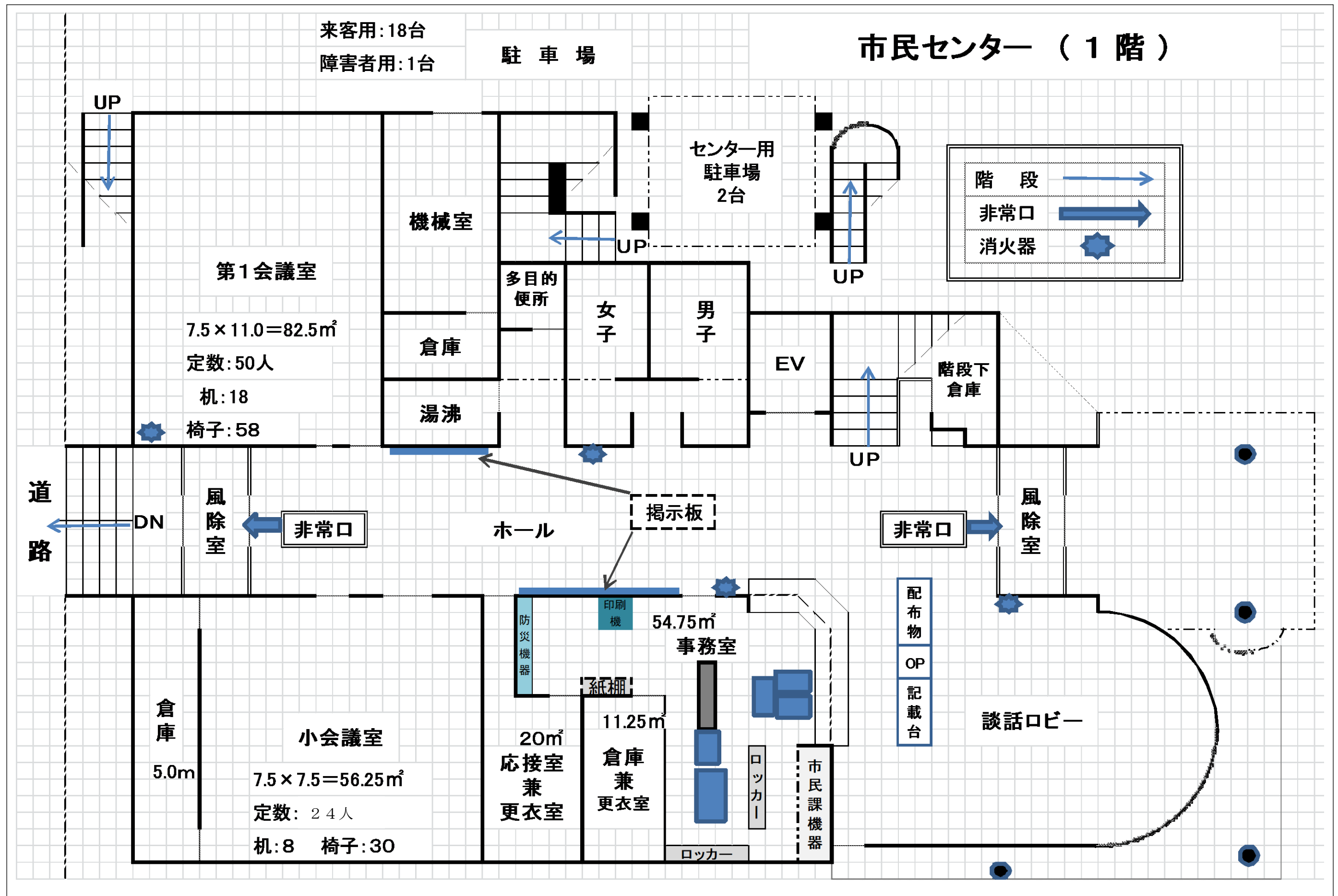
市民センター1階平面図
