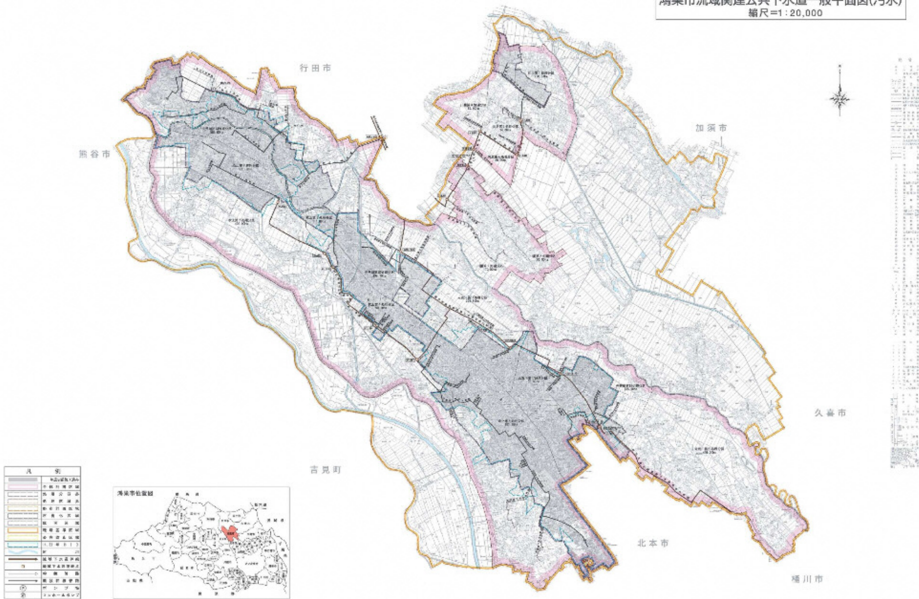
図 2 鴻巣市の下水道計画一般図(汚水)
