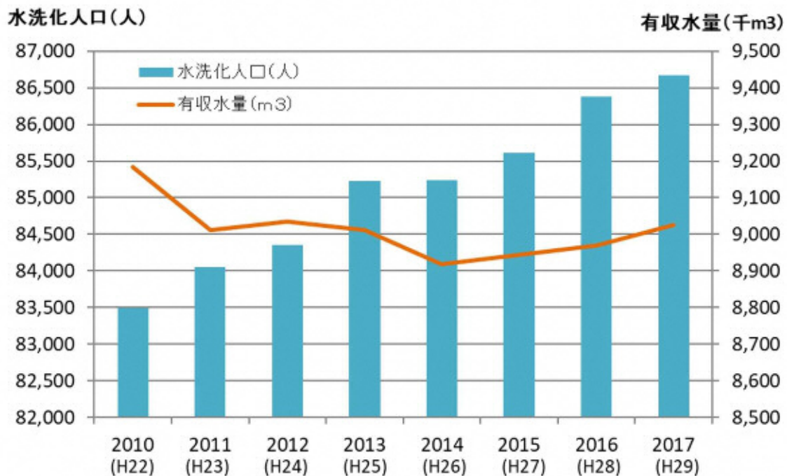
図 5 水洗化人口と有収水量の推移
